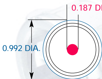
1/4" MINI TC
