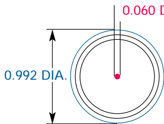
1/8" MINI TC
